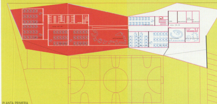
PLANTA PRIMERA
